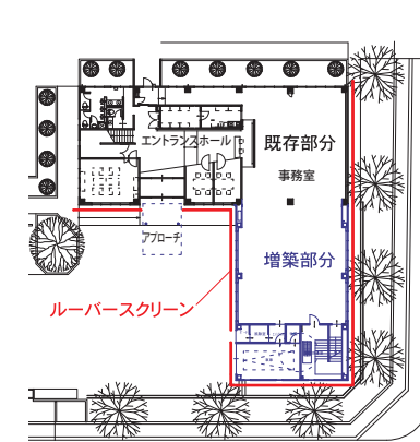
1階平面図 S:1/750
