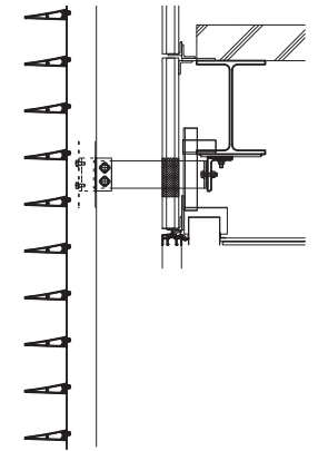
ルーバースクリーン部分断面図 S:1/30
